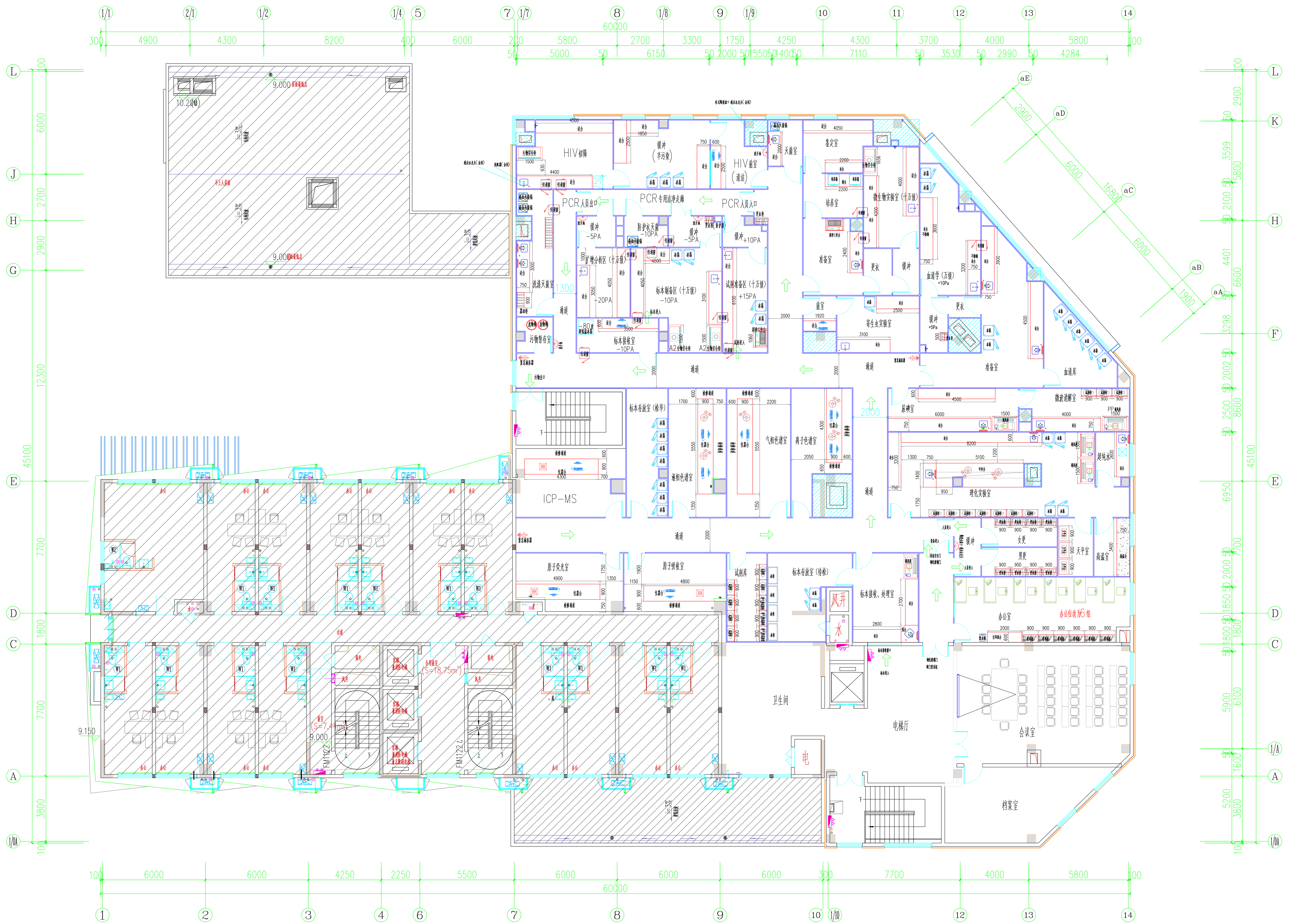
B-S1 #楼三层平面规划布置图
